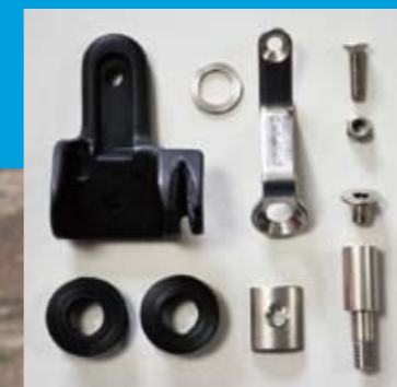
POWER Q6 クリート
